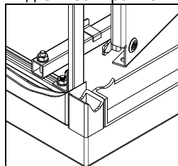
Вид С – Запирание внизу
