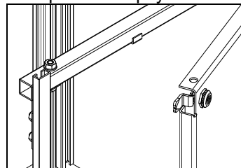
Вид А – Запирание сверху
