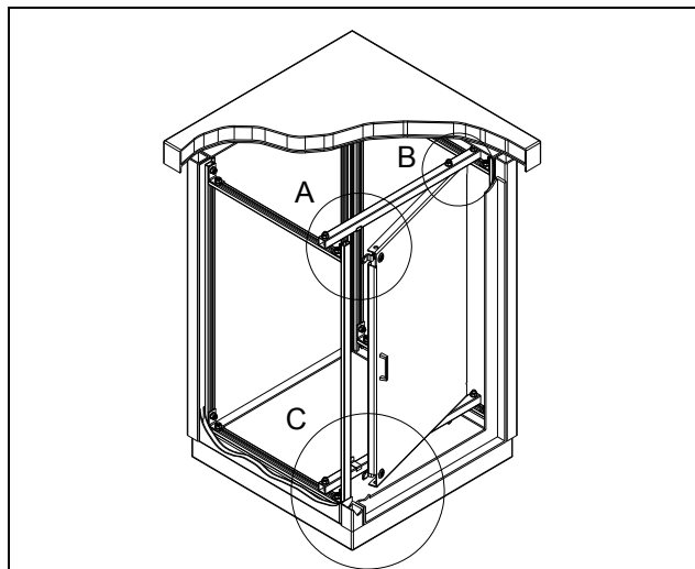
(Шкаф, изображённый в частичном разрезе)
