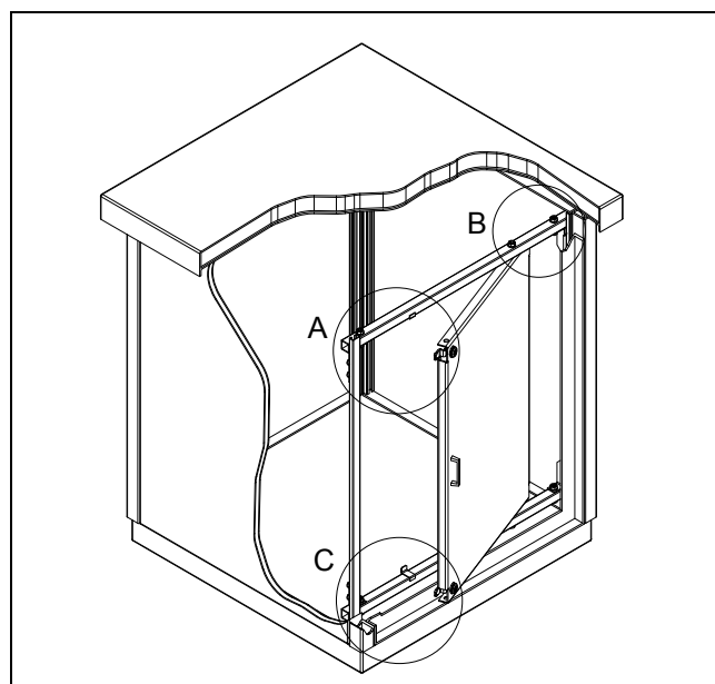
(Шкаф, изображённый в частичном разрезе)
