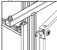
Вид С – Запирание внизу
