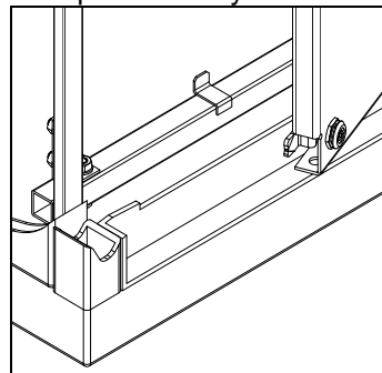
Вид С – Запирание внизу
